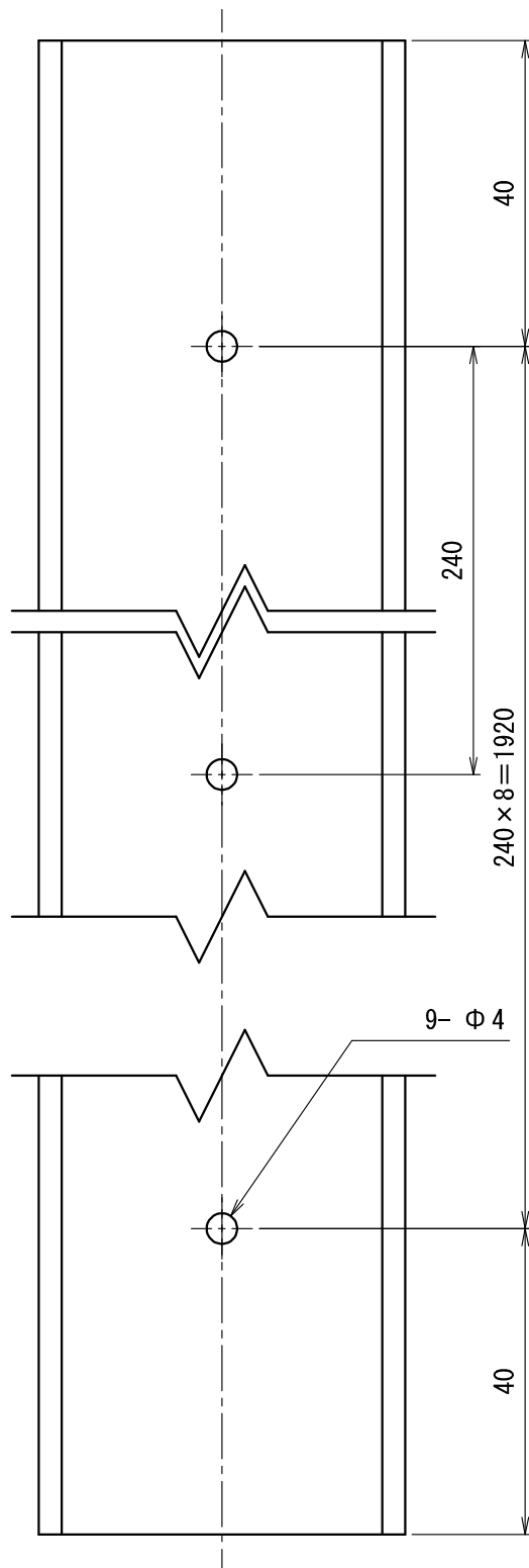
製品裏面穴詳細
